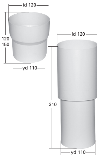
Forhøyningstuss for WC til plast og N-rørs muffe
