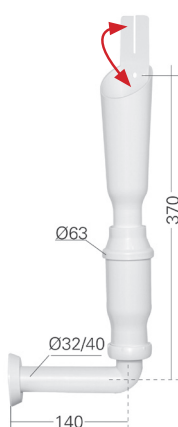
Vinklet vannlås med vaskemaskin-trakt
