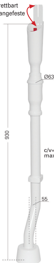
Rettt vannlås for gulvtilslutning
