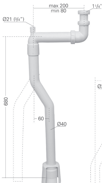
FlexiGulv NRF 451 7003 Art.nr 45830 40 mm
