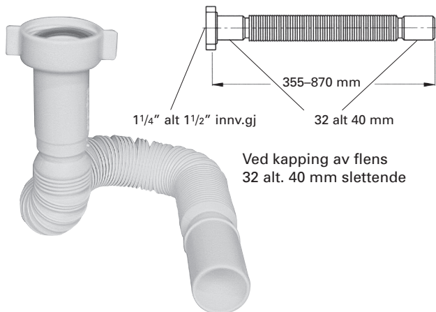
Fleksibel avløpsslange, lengde 355–870 mm
