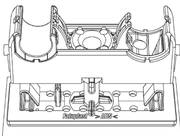
Bilde 2. Monter rørklammerunderdel på limplaten.
