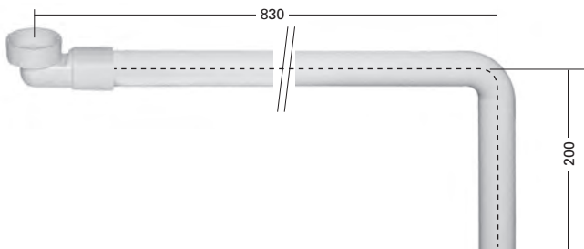
Kylpyammeen poistoputki 200 x 830 mm kulmayhteellä 1 1/4" - 1 1/2" ja kumitiivisteellä
