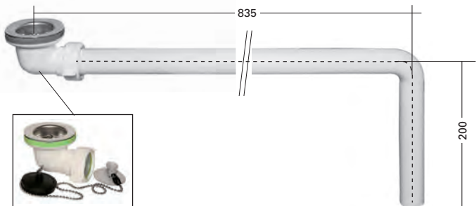
Poistoputki 200 x 835 mm kulmaventtiilillä
