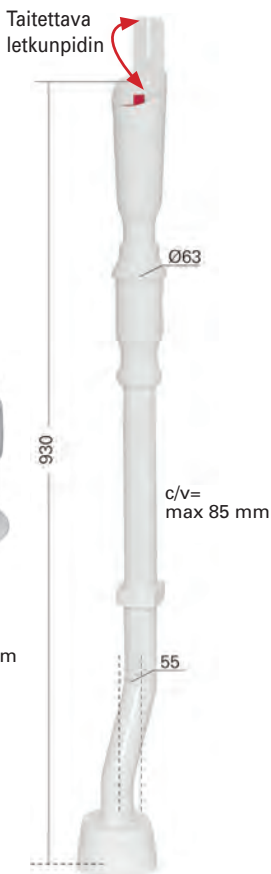
V-lukko lattialiitännällä LVI
