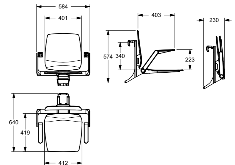
Ascento Einhängesitz klappbar, mit Rückenlehne und Armlehnen Code PG 8700 Ascento Suspendable lift-up seat, with backrest and armrest
