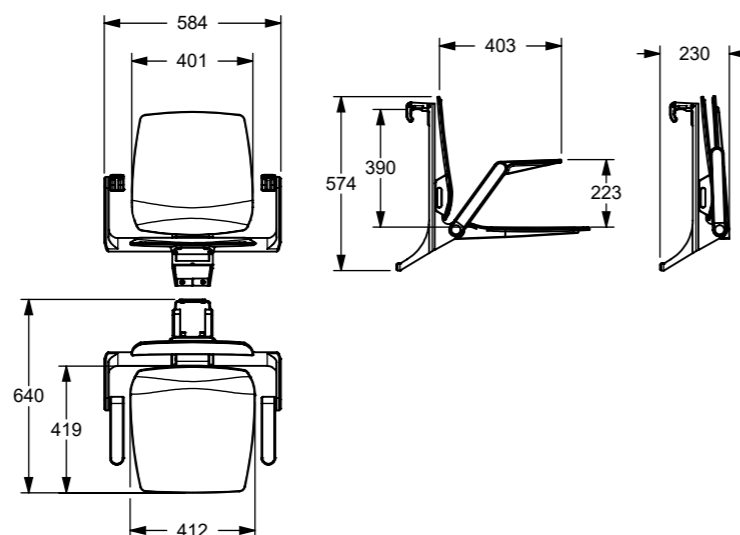
Ascento Einhängesitz klappbar, mit Rückenlehne und Armlehnen Code PG 8700 Ascento Suspendable lift-up seat, with backrest and armrest
